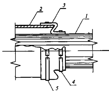
1 — трубная плетка, 2 — защитный футляр, 3 — резиновая манжета, 4 — малый комут, 5 — большой комут
