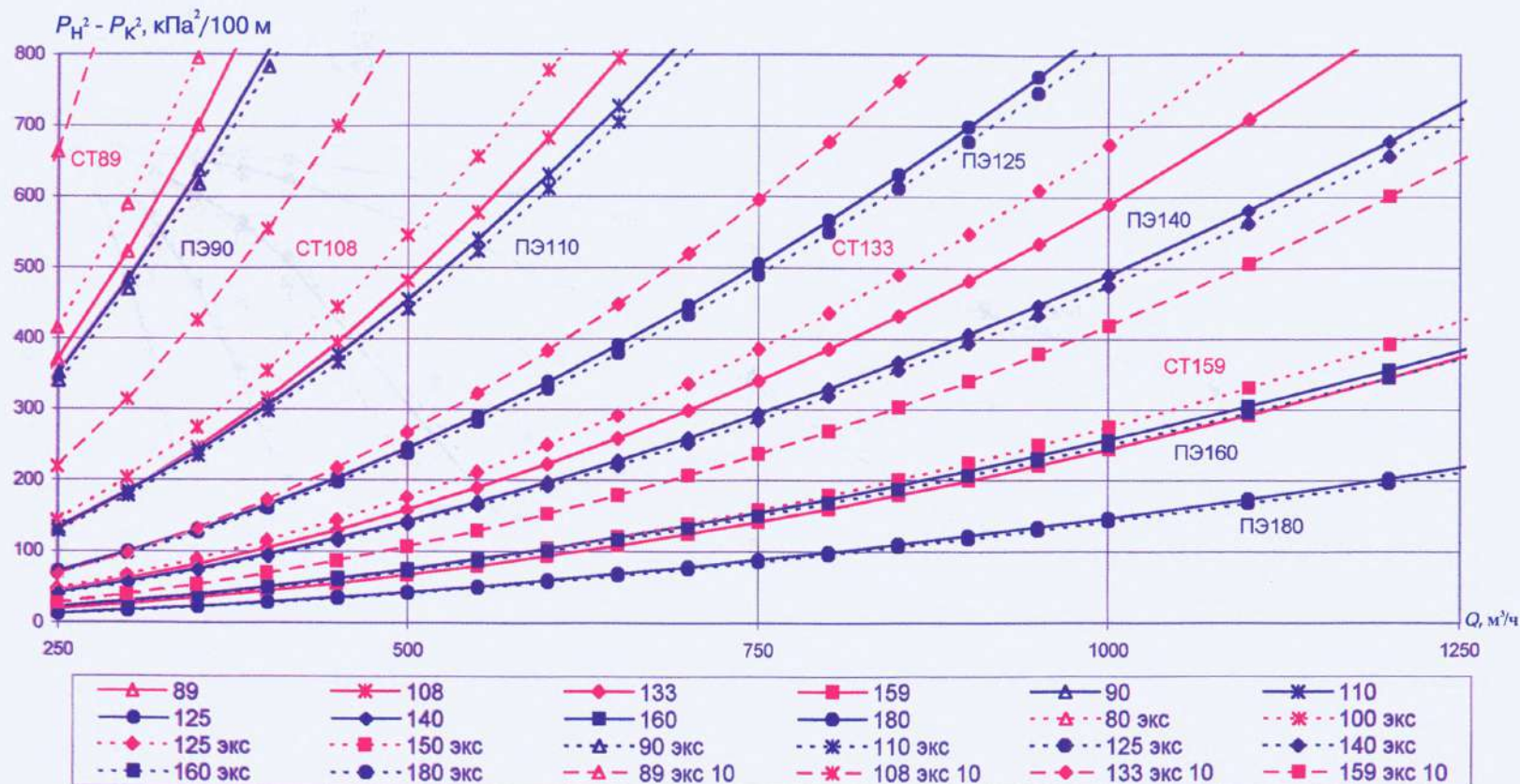
Удельные потери давления для стальных и полиэтиленовых труб (новых и бывших в эксплуатации) низкого давления ( Q 250 - 1250 м 3 /ч, \rho = 0,73 кг/м 3 , \nu = 1,4 \times 10^{-6} м 2 /с)
