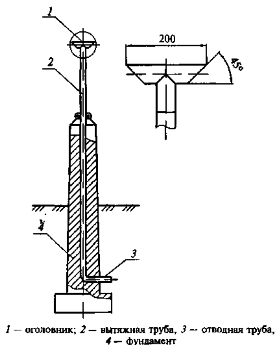
Рисунок 2 — Вытяжная свеча
