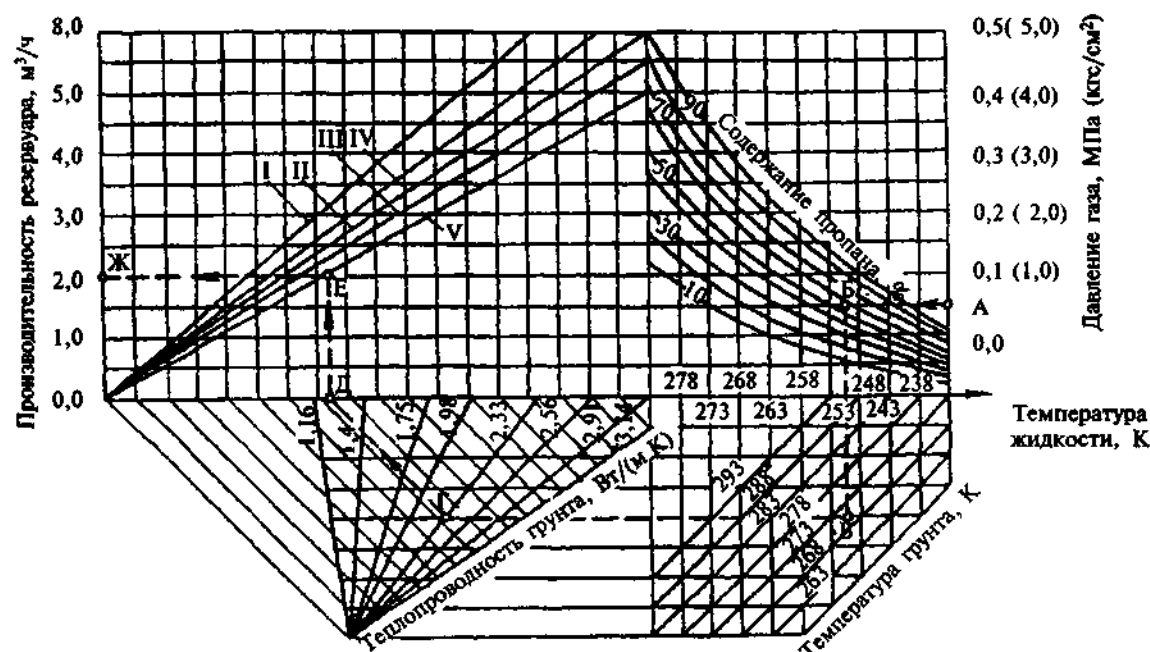
Рисунок 7 — Номограмма для определения производительности резервуара сжиженного газа вместимостью 2,5 и 5 м³ (подземного)
