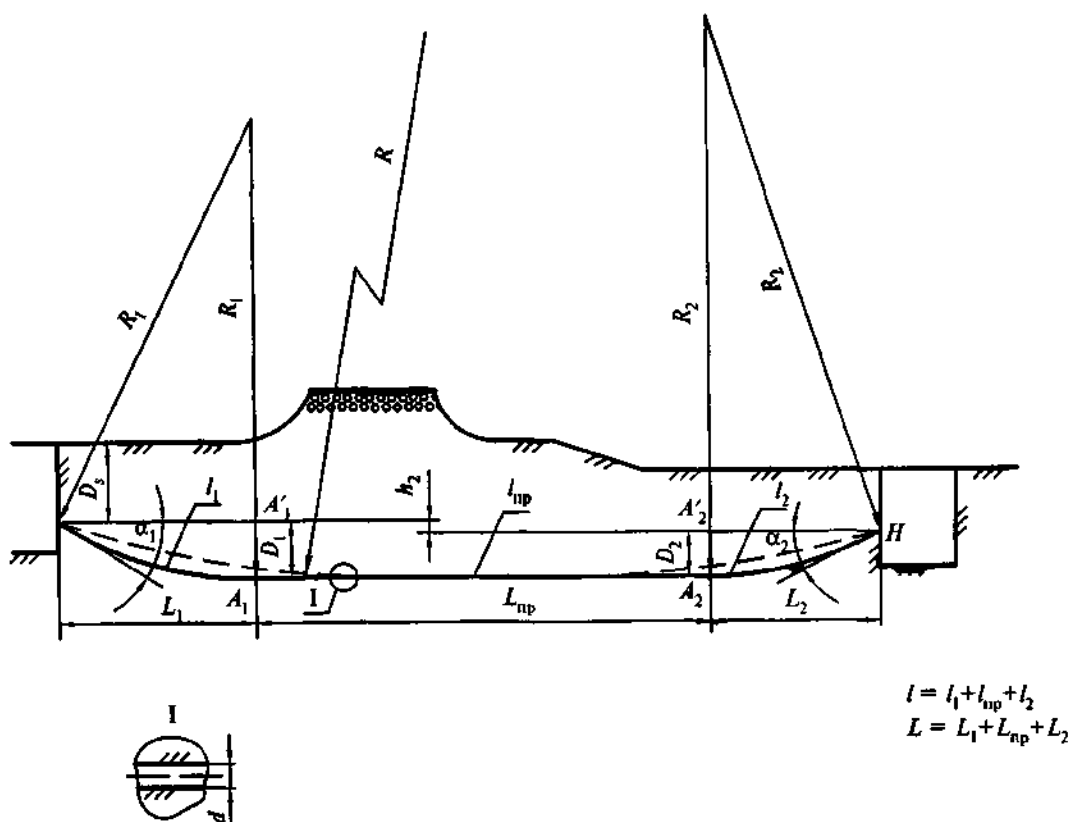
Рисунок Л.1 — Основные геометрические параметры трассы
