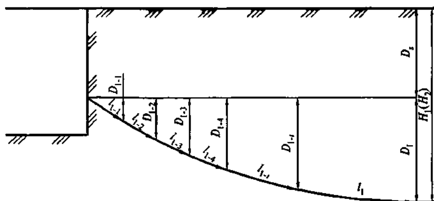
Рисунок Л.3 — Схема перехода пилотной скважины от максимального угла забурирования к нулевому углу
