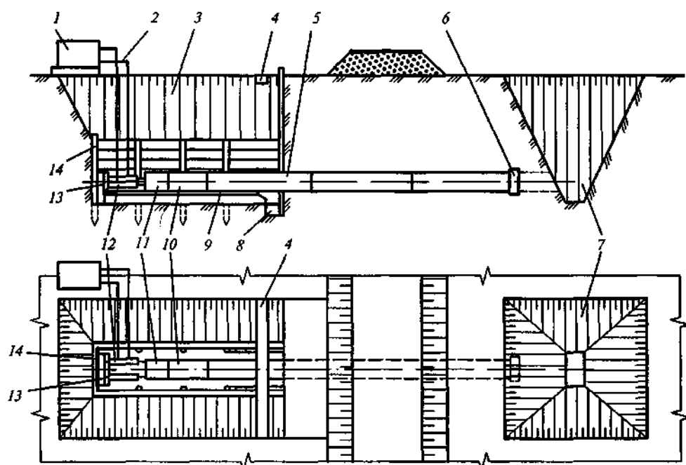
1 — насосная станция, 2 — газопровод, 3 — рабочий котлован, 4 — водоотводный лоток, 5 — защитный футляр, 6 — лобовая обделка (нож), 7 — приемный котлован, 8 — приямок для сварки защитного футляра, 9 — направляющая рама, 10 — нажимной патрубок, 11 — нажимная заглушка, 12 — гидродомкраты, 13 — башмак, 14 — упорная стенка
