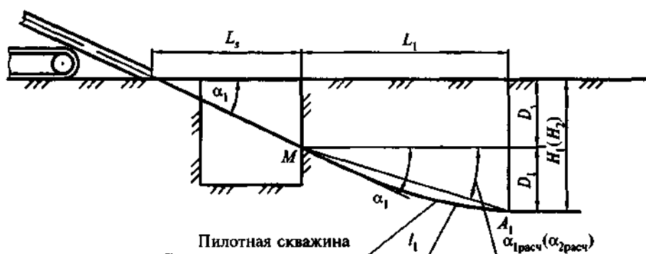
Рисунок Л.2 — Схема забурирования пилотной скважины
